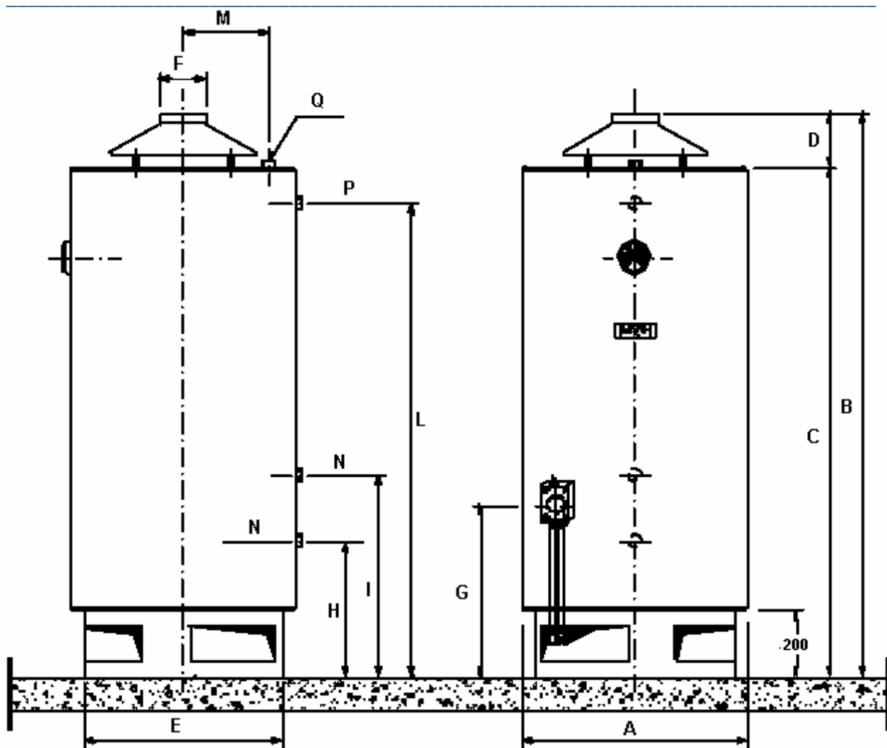
Рис. 3. Размеры водонагревателя
